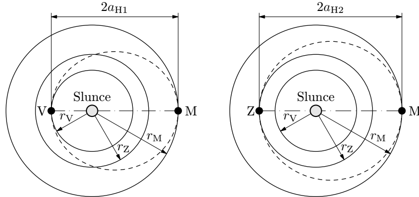
Obr. R1 Mars – Venuše
